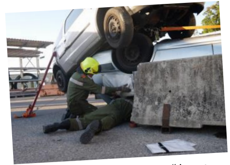
Einstieg des „Inneren Retters“ in am Dach liegendes Unfallfahrzeug
